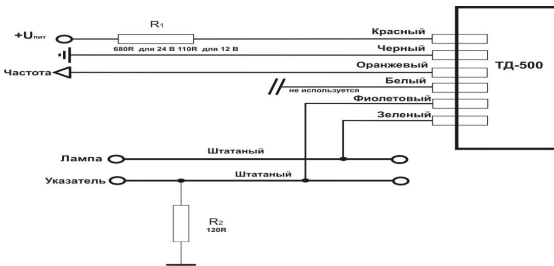
Рис. 13 Схема включения в частотном режиме.
